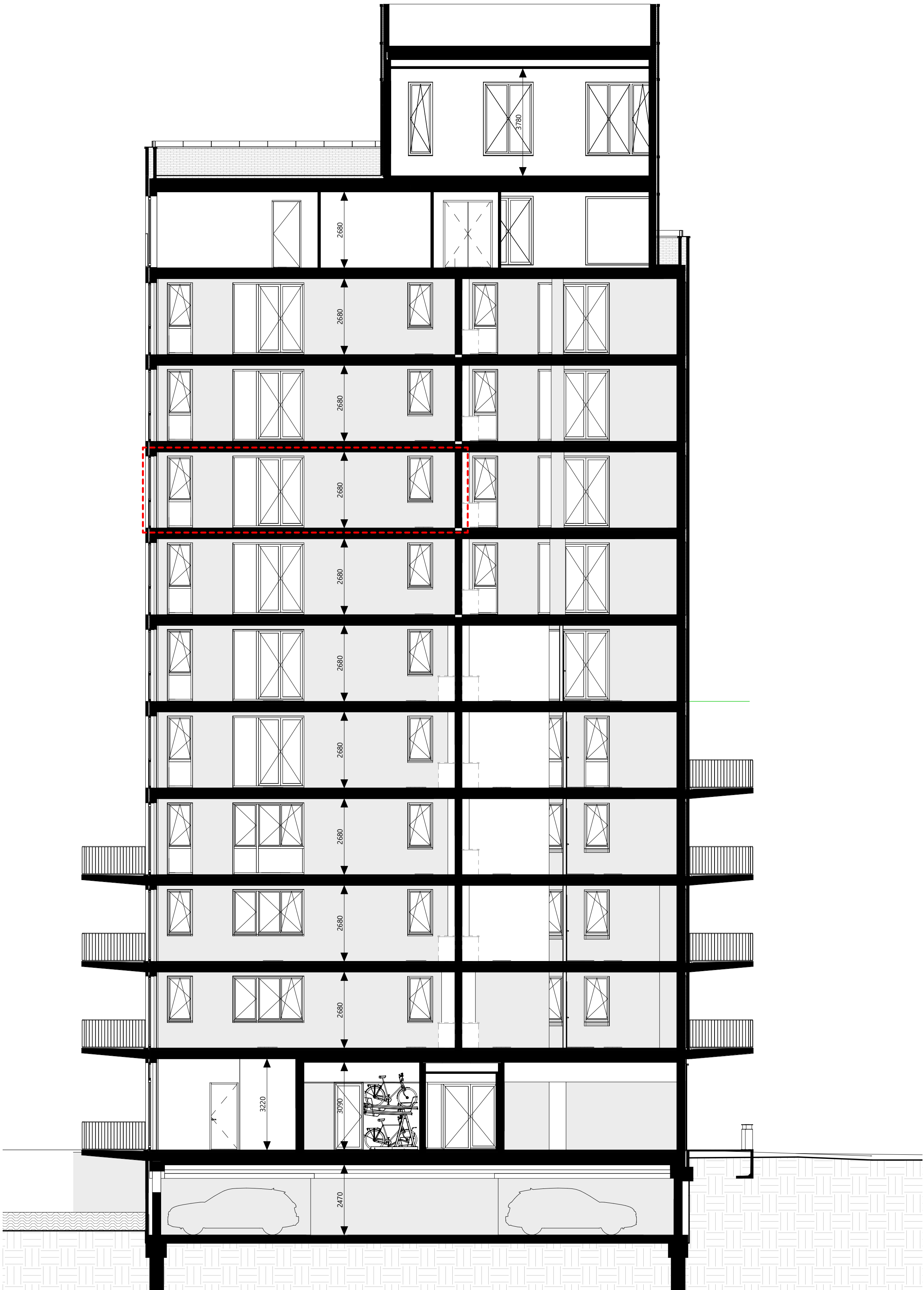
doorsnede B 1 : 100
