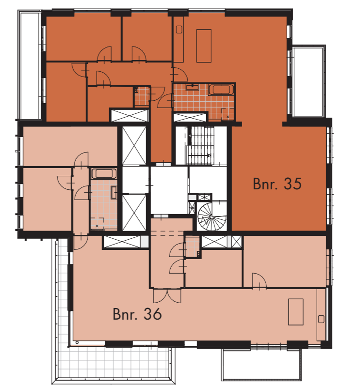
TIENDE VERDIEPING
