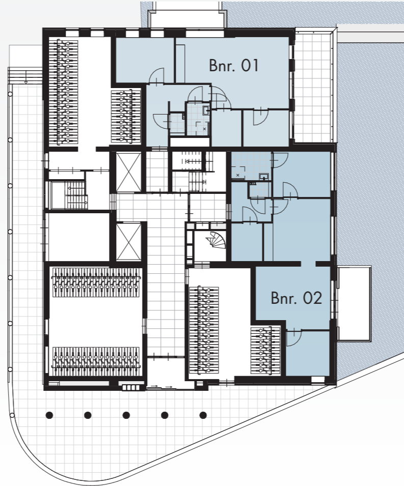
BEGANE GROND
