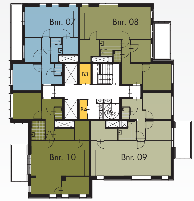
TWEEDE VERDIEPING
