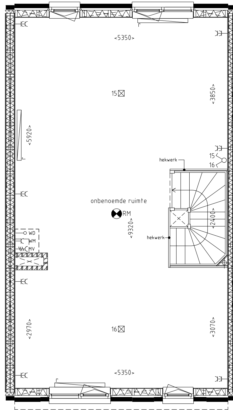
2e verdieping
