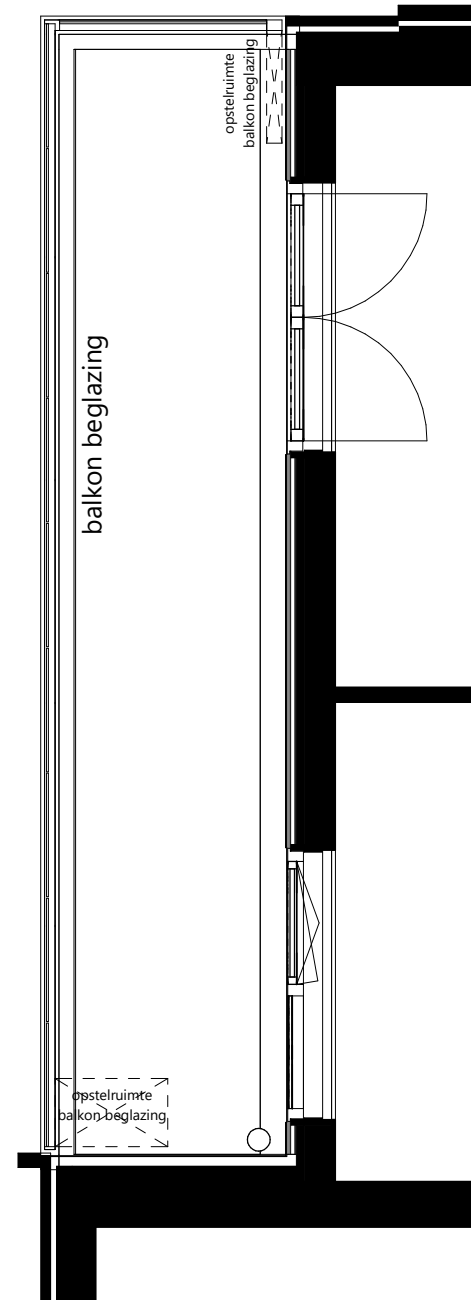
plattegrond 1 : 50
